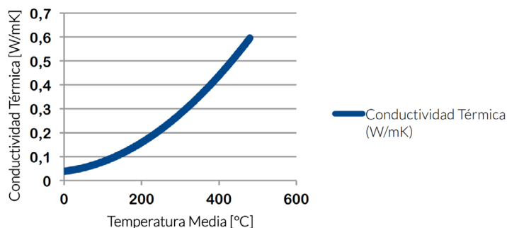
Conductividad térmica vidrio celular
